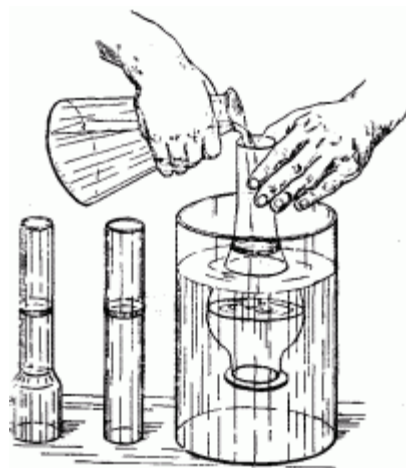
Рис. 54. Давление жидкости на дно сосуда зависит только от площади дна и от высоты уровня жидкости. На рисунке показано, как проверить это правило.
