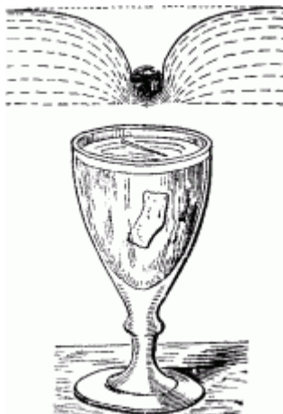
Рис. 61. Игла, плавающая на воде. Вверху – разрез иглы (2 мм толщины) и точная форма углубления на воде (увеличено в 2 раза). Внизу – способ заставить иглу плавать на воде с помощью лоскутка бумаги.
