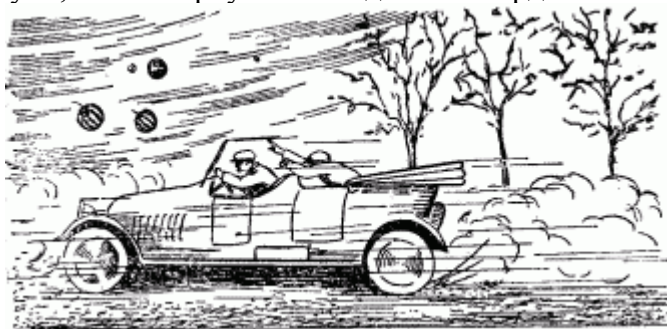
Рис. 21. Арбуз, брошенный навстречу быстро мчащемуся автомобилю, превращается в “снаряд”.
