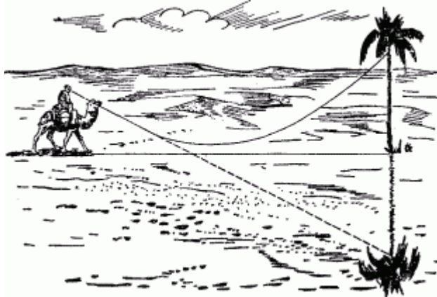
Рис. 115. Как возникает мираж в пустыне. Этот рисунок, обычно воспроизводимый в учебниках, представляет путь светового луча наклоненным к земле преувеличенно круто.
