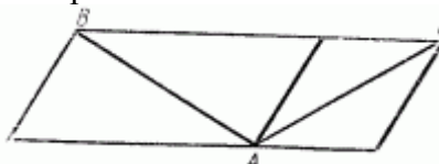
Рис. 144. Расстояния АВ и АС равны, хотя первое кажется больше.
