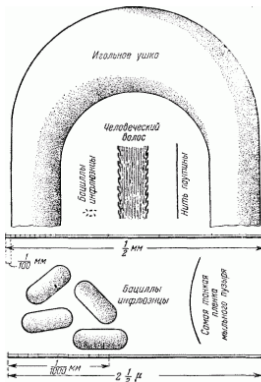
Рис. 69. Вверху – игольное ушко, человеческий волос, бацилла и паутинная нить, увеличенные в 200 раз. Внизу – бациллы и толщина мыльной пленки, увеличенные в 40000 раз. 1 мю=0,0001 см.
