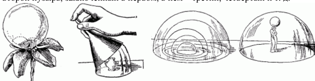
Рис. 66. Опыты с мыльными пузырями: пузырь на цветке; пузырь вокруг вазы; ряд пузырей друг в друге; пузырь на статуэтке внутри другого пузыря.
