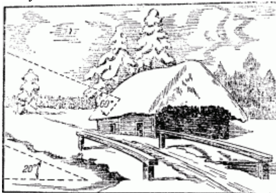
Рис. 87. Лучи Солнца греют наклонную крышу сильнее, чем горизонтальную земную поверхность (числа указывают величину углов).
